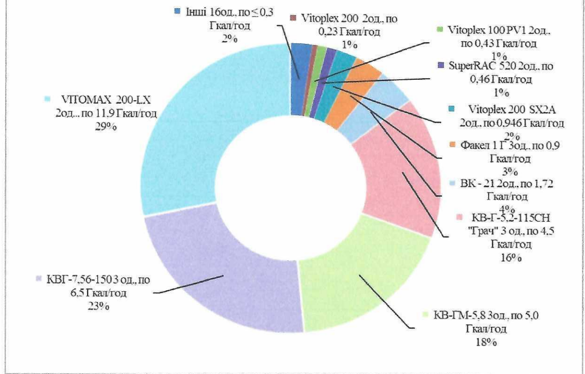
Рис.1. Розподіл установленної потужності за типами котлоагрегатів
